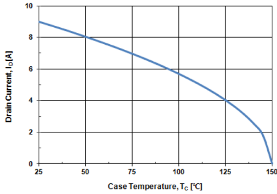
Fig. 9 I_D - T_C
