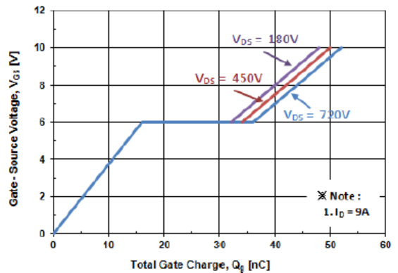
Fig. 6 V_{GS} - Q_G
