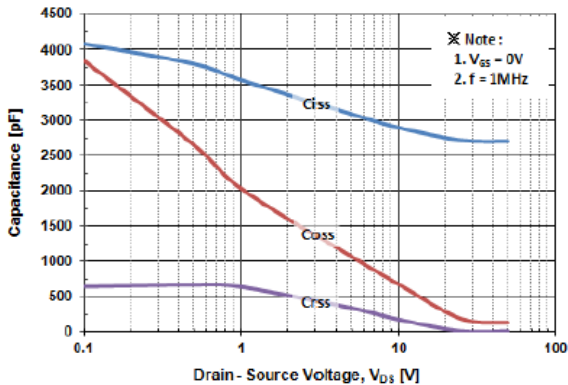
Fig. 5 Capacitance - V_{DS}
