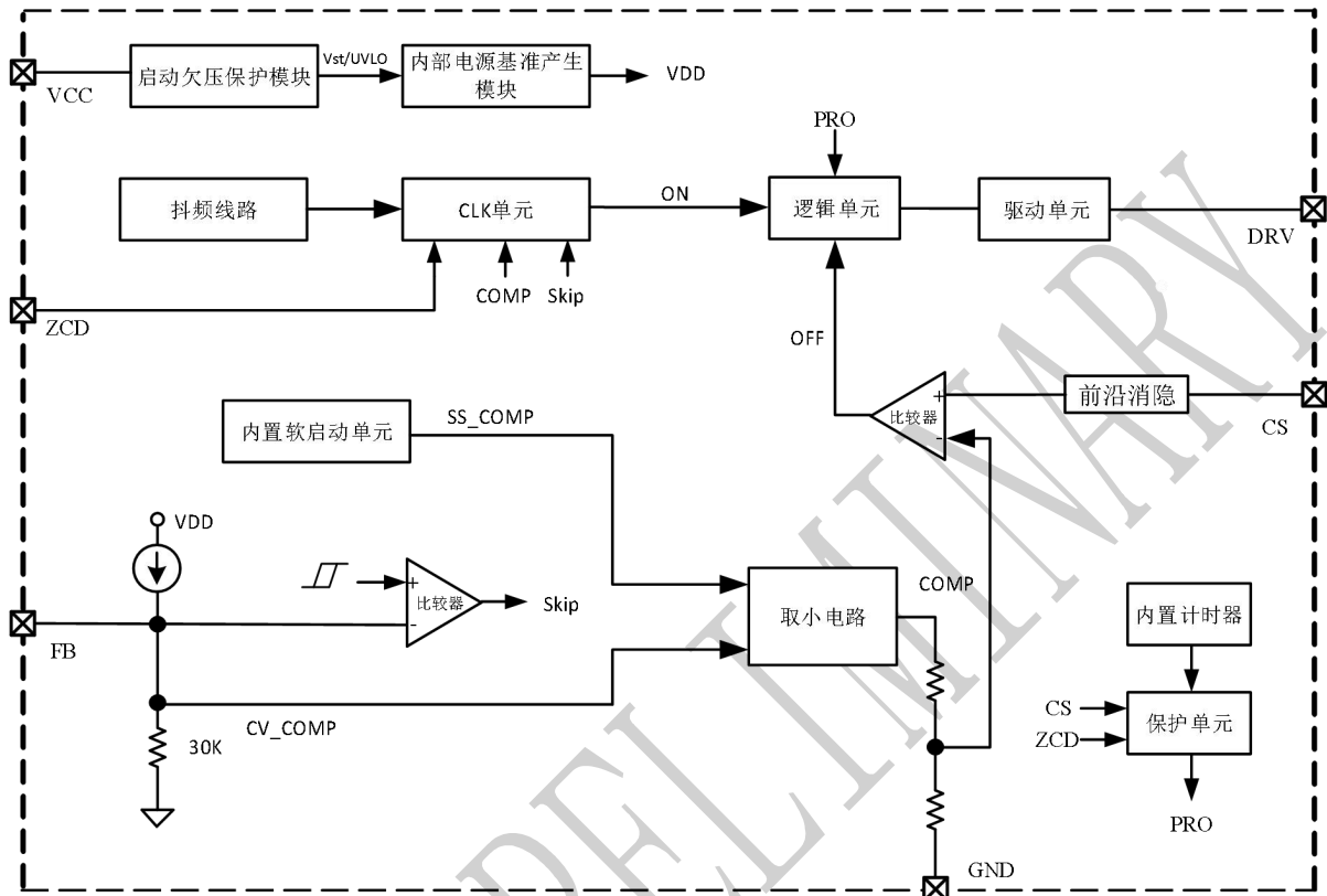
图3 LP8841SC 内部框图
