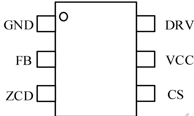
图 2 管脚封装图
