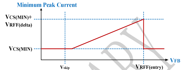
图 5 MPCM 模式
