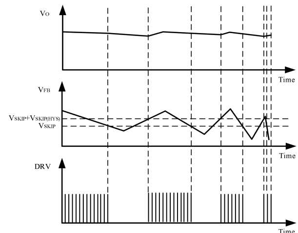
图 6 打嗝模式
