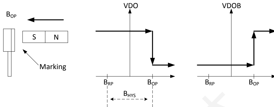
图 5 磁场特性图
