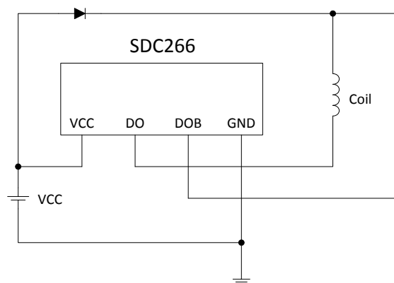
图 7. 典型应用图
