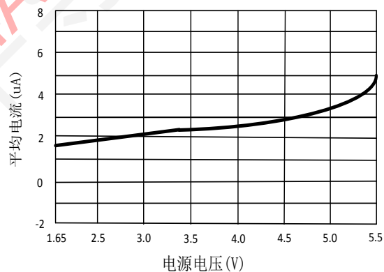
图 5. 平均电流 VS 电源电压 ( T_a=25^{\circ}C )
