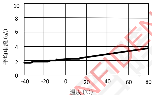
图 4. 平均电流 VS 环境温度 ( V_{DD}=3.3V )
