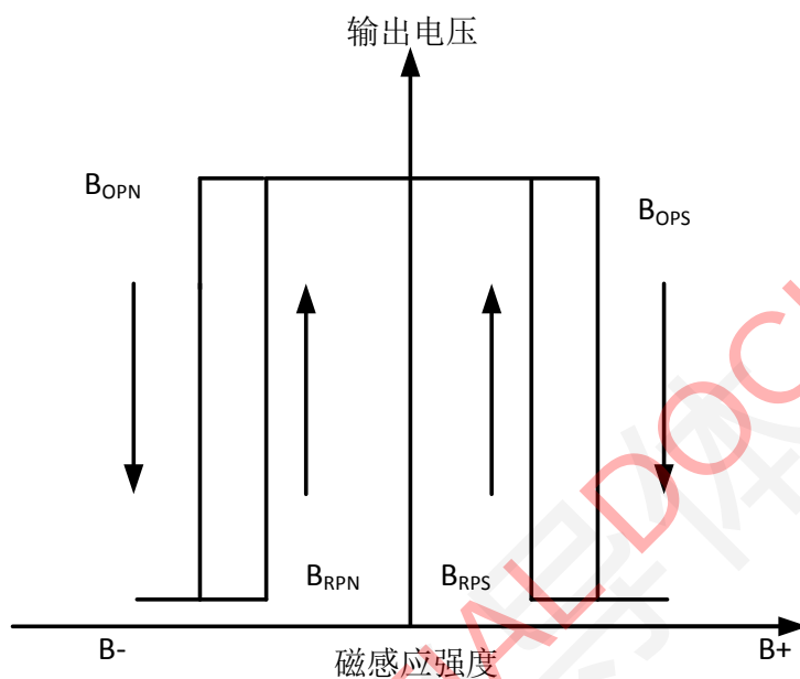
图 6. 磁场特性图
