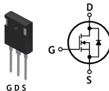
TO-247-3L
